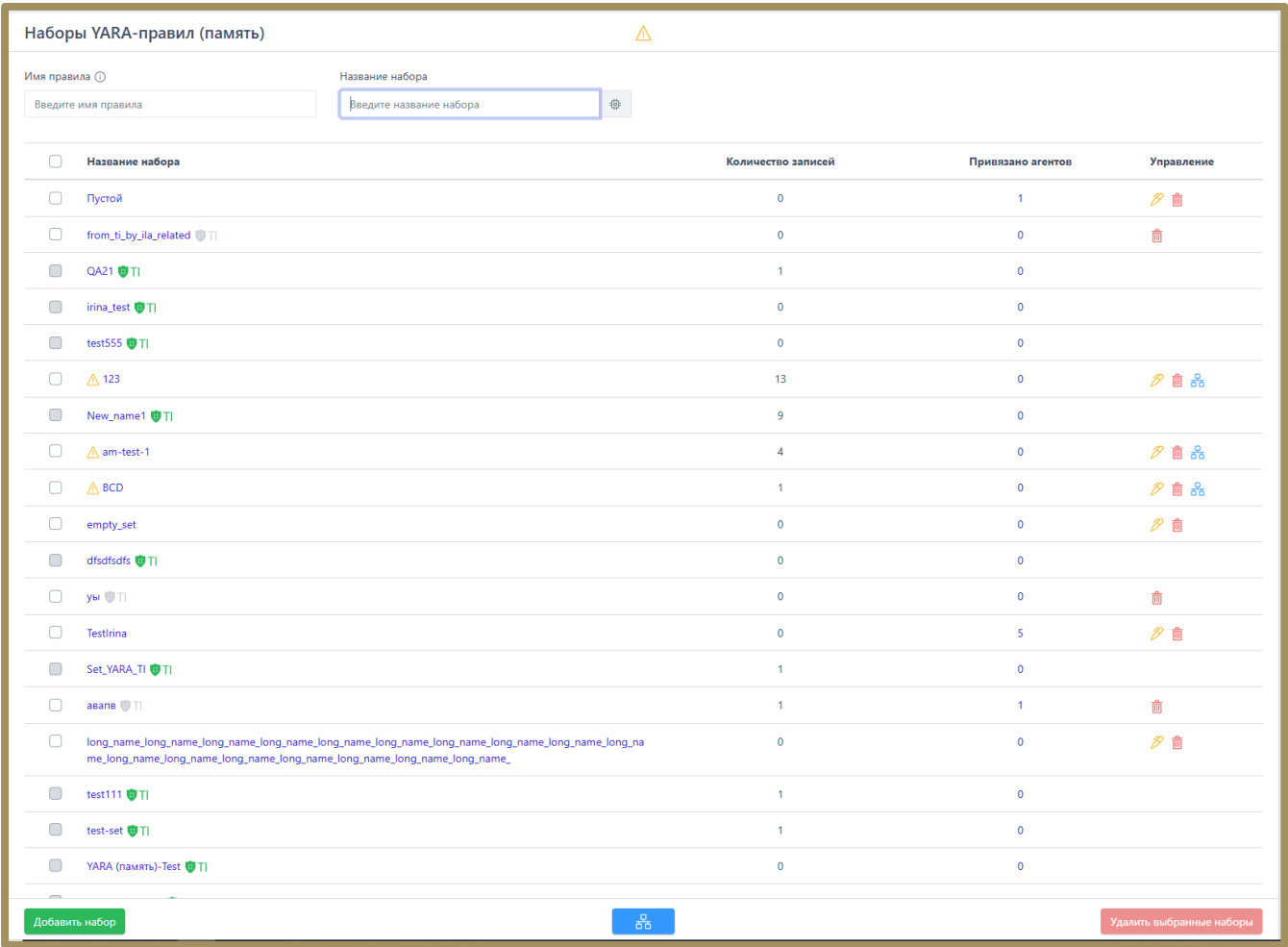
Рисунок 47 – YARA-правила (память)
