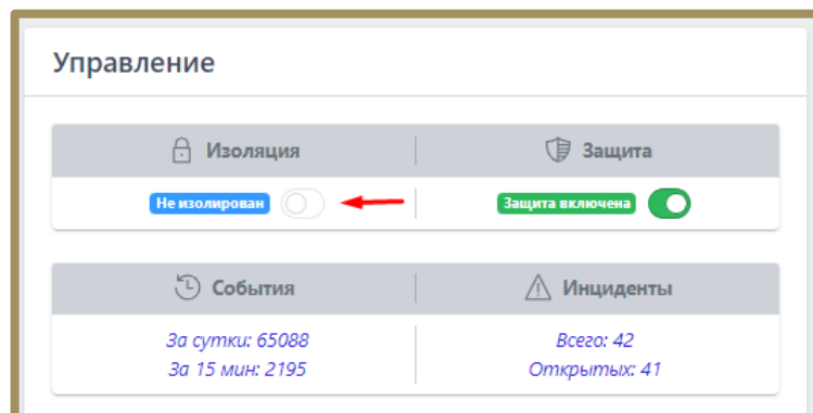
Рисунок 73 – Изоляция агента
