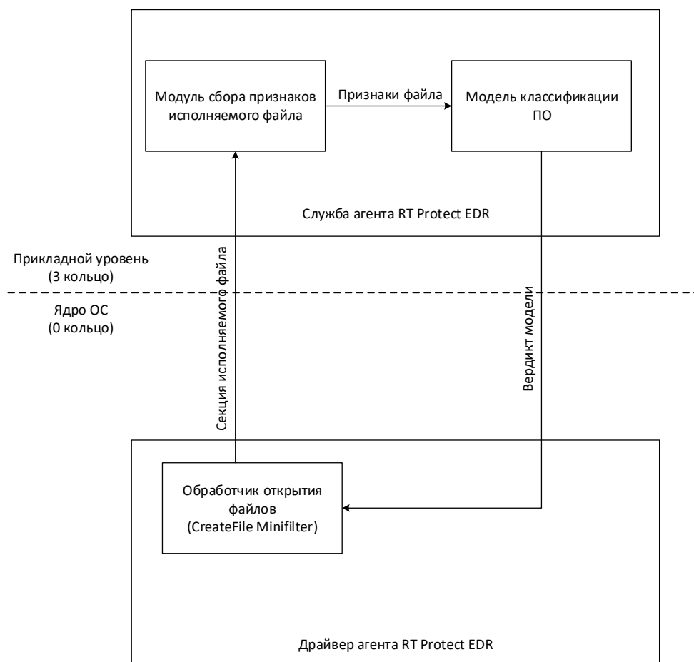
Рисунок 99 – Схема применения модели классификации ПО
